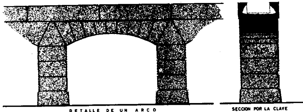
ACUEDUCTO ROMANO DE ALBATANA Escala en metros 0 0'25 0'50 0'75 1'00 1'25 1'50 1'75 2 ALBACETE MARZO 1975
