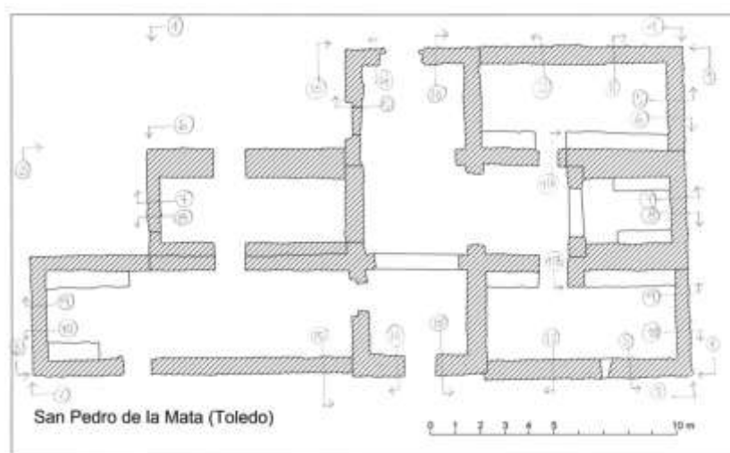
Vista desde el lado Noroeste (camino) y el plano de la planta de S. Pedro de la Mata (Toledo), extraído del proyecto de investigación 2016 denominado: “Arqueología de la arquitectura en la Iglesia de S. Pedro de la Mata (fase II)”, dirigido por D. Jose Manuel Baltuille Martín.
