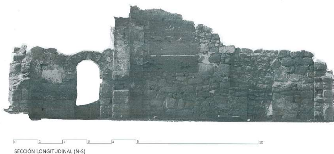
Sección longitudinal (N-S) del yacimiento de S. Pedro de la Mata (Sonseca-Toledo). Imagen extraída del proyecto de investigación 2016 denominado: “Arqueología de la arquitectura en la Iglesia de S. Pedro de la Mata (fase II)”, dirigido por D. Jose Manuel Baltuille Martín.
